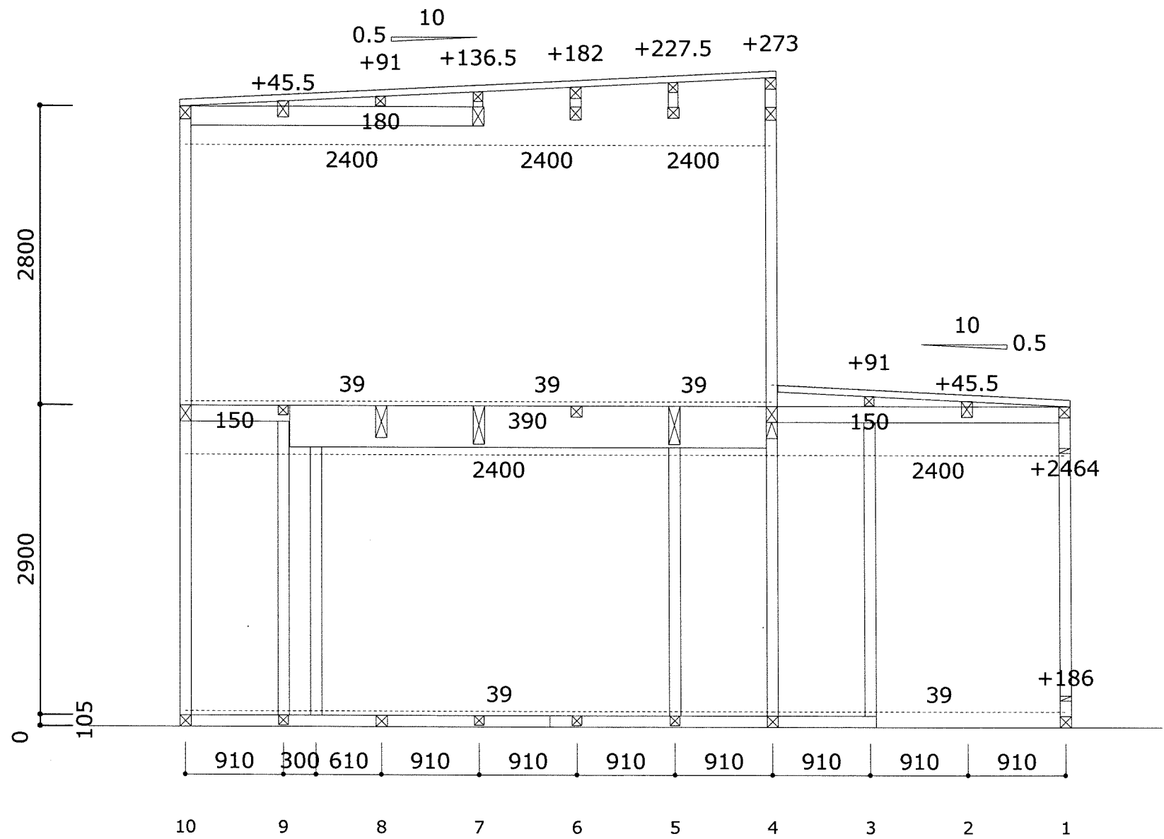
ほ通り 東面
