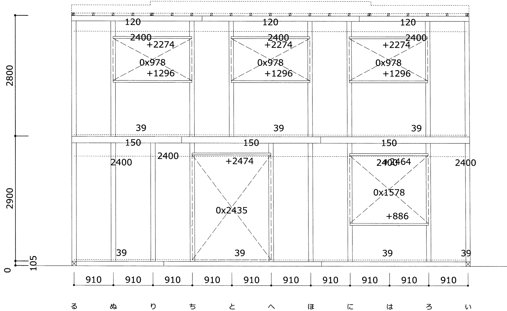
10通り 南面
